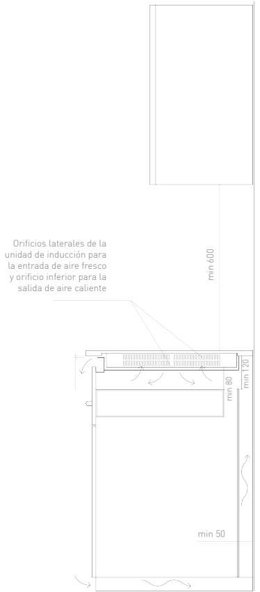
Img.2: Distancias mínimas de los armarios
