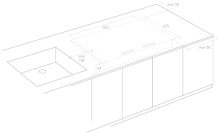
Abb.1: Abmessungen des Induktionsherdes und Mindestabstände zum Arbeitsplattenrand
